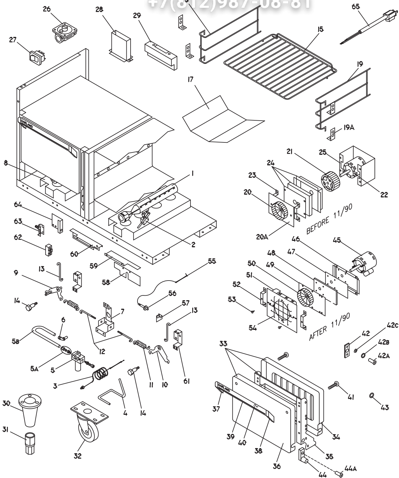
HP280-Oven Section.dwg
