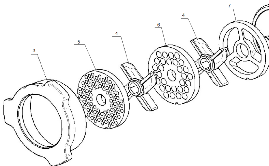
Рисунок 1 Мясорубка МЭП-300
