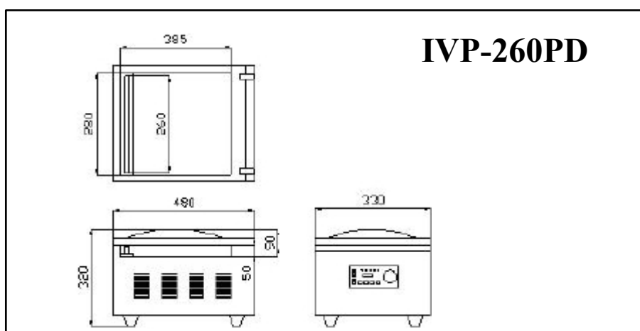
Рисунок 4.7 – Размеры вакуумного упаковщика модели IVP-260PD
