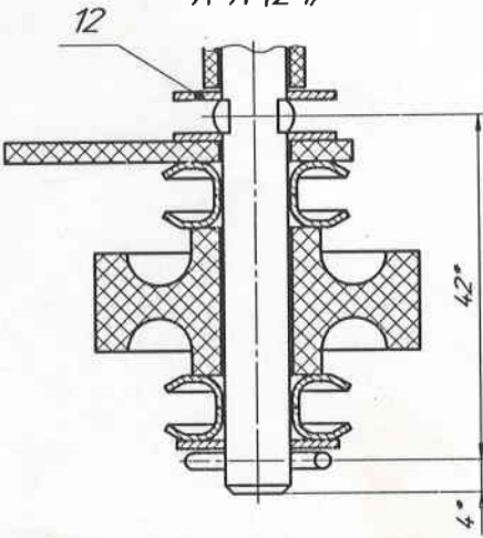
А-А (2:1)
