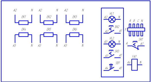
Рисунок 2 – схема электрическая принципиальная шкафов ШЖЗ-01
