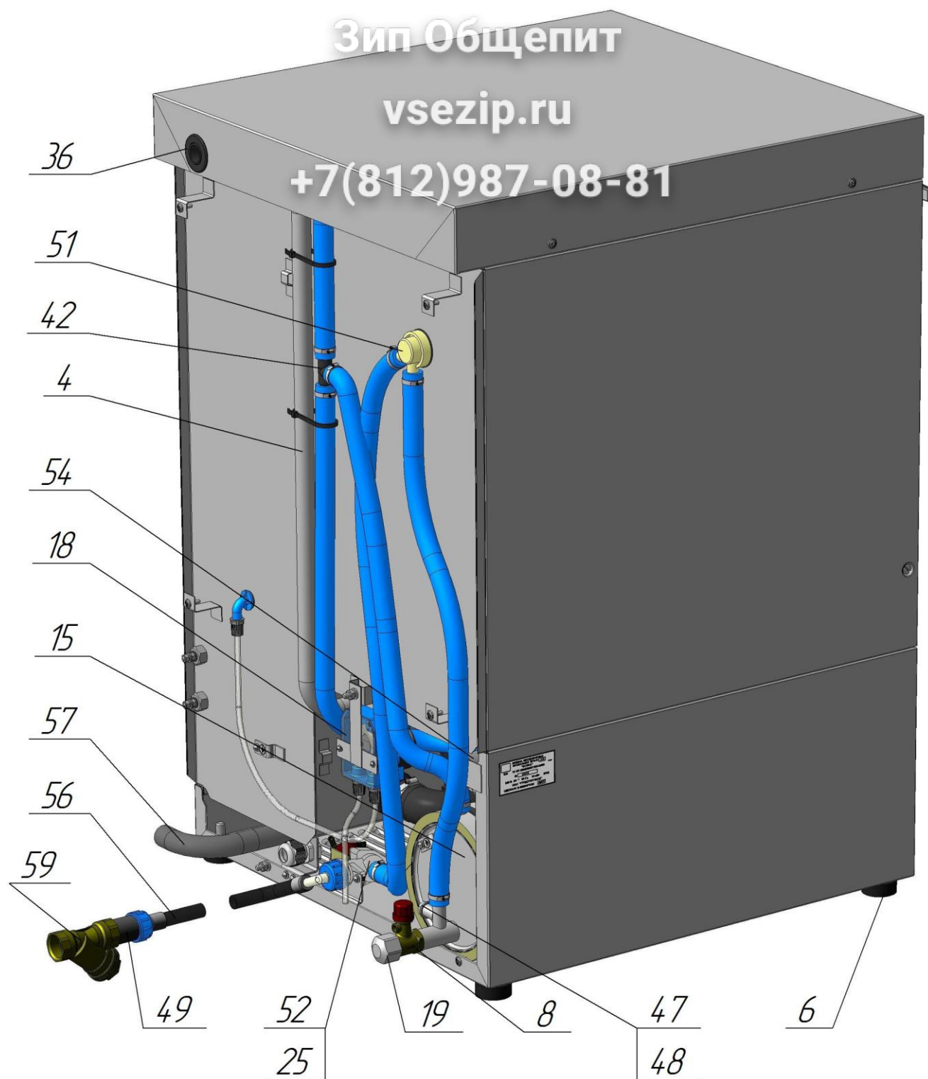
Рисунок 3. Машины посудомоечные фронтальные МПФ-12-01 "Котра" и МПФ-30-01 "Котра" (вид сзади)
