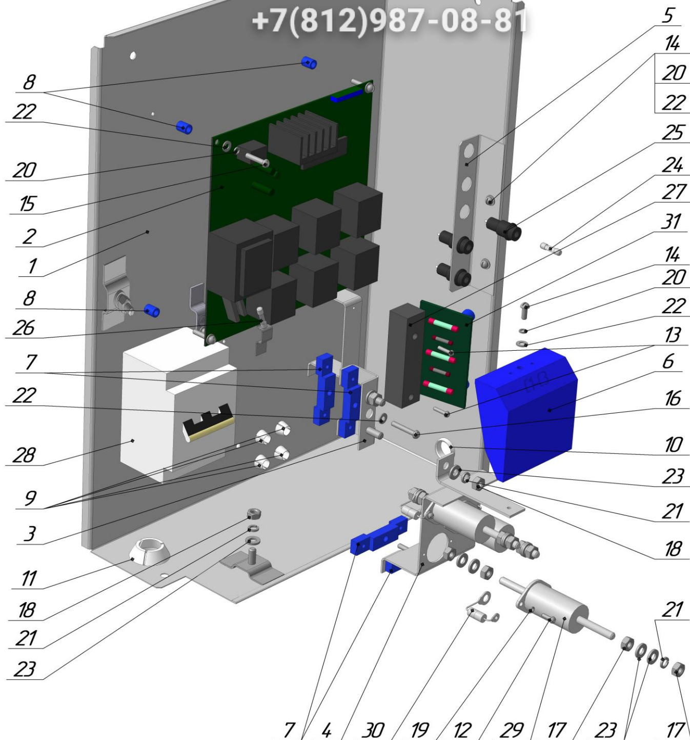
Рисунок 6 – Электрошкаф МПУ-700 01.17.000
