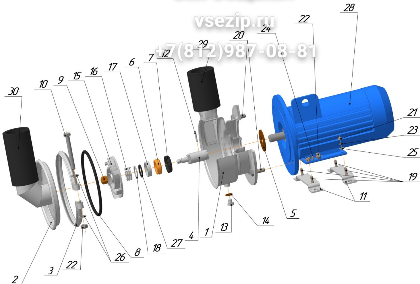
Рисунок 4 – Электронасос МПУ-700 01.04.000
