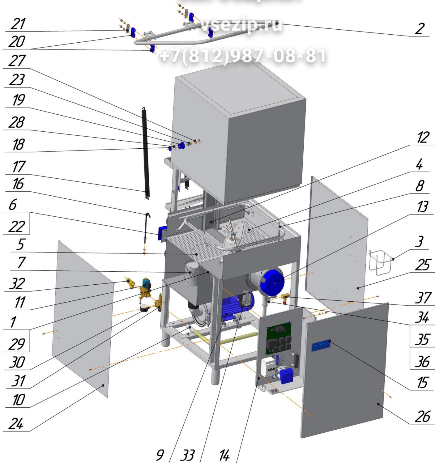
Рисунок 2 – Секция мытья МПУ-700 01.00.000-01
