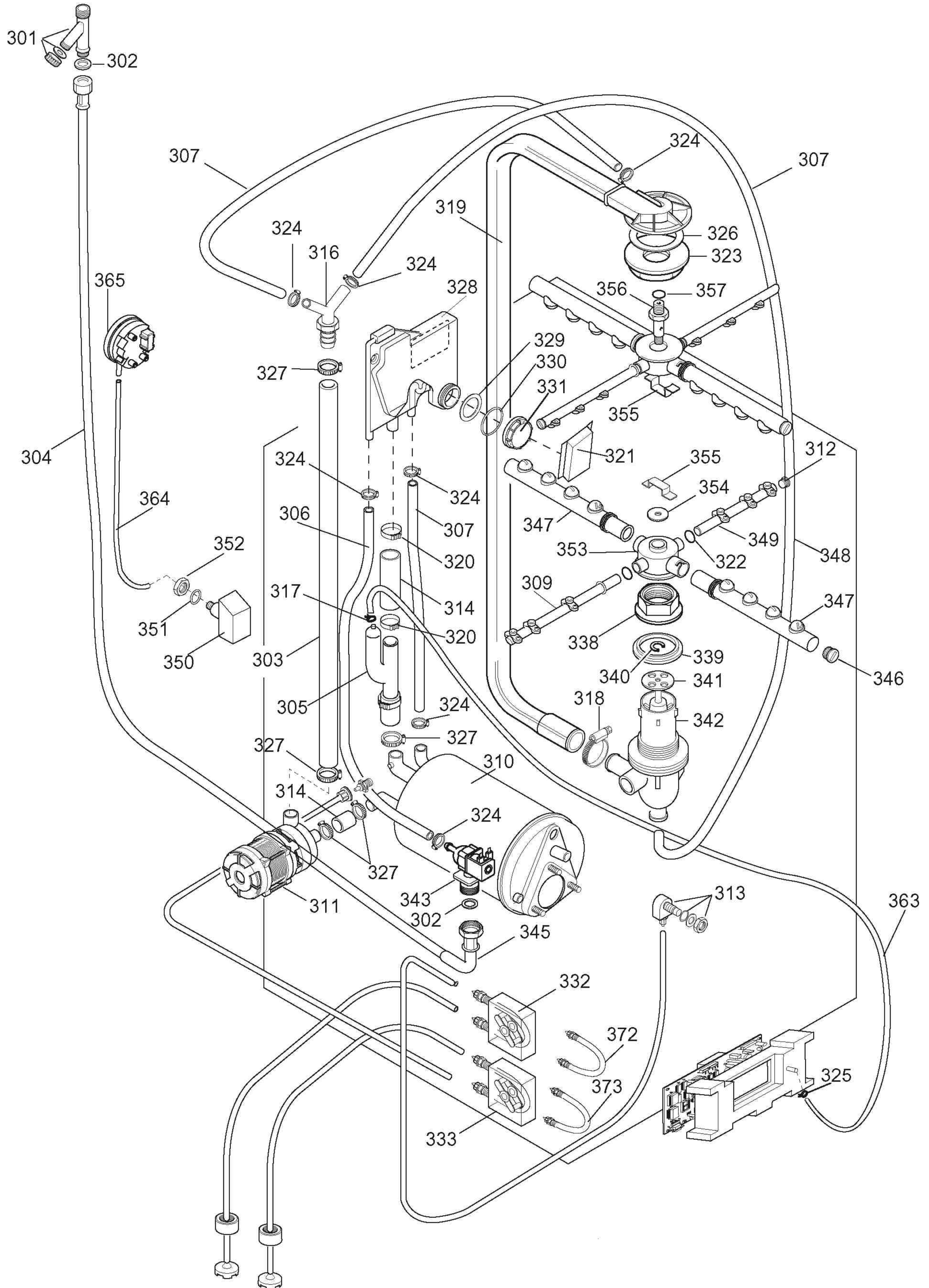
ил. 611002p4 Circuito idraulico / Hydraulic circuit
