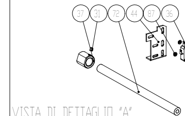
VISTA DI DETTAGLIO "A"
