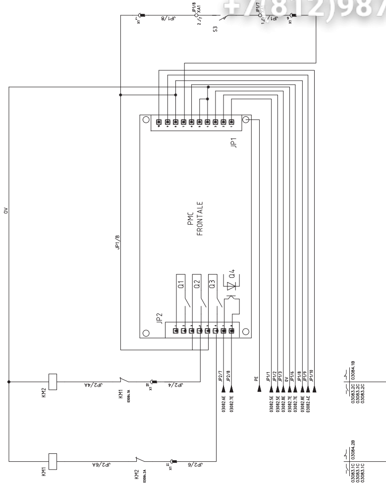
FIG. / ПИС. 29 - MX40/60/80 EV Schema elettrico / Electrical diagram / Schemas électriques / Diagrama eléctricos / Монтажная схема
