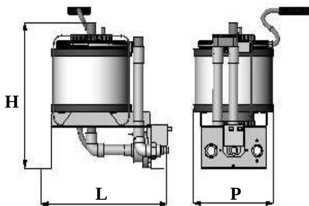
GRUPPO VAPORIZZATORE
