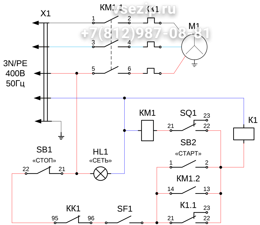
Зип.Общедит Схема электрическая принципиальная МКО-50
