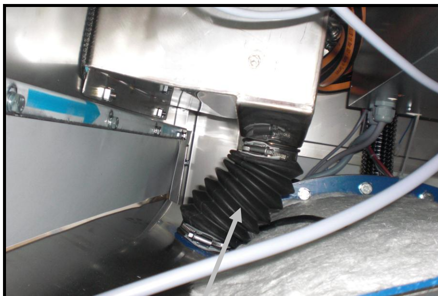
Faltenbalg / bellows Pos. 18
