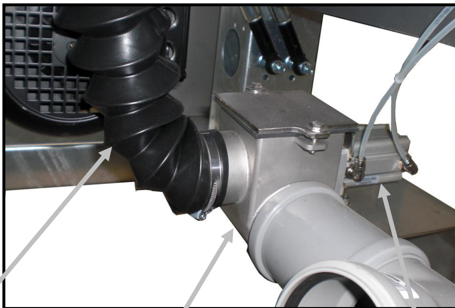
Ablaufventil / drain valve Pos. 29
