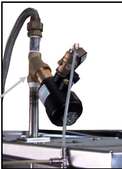
Bild: Dampfbeheizung / picture: steam heating
