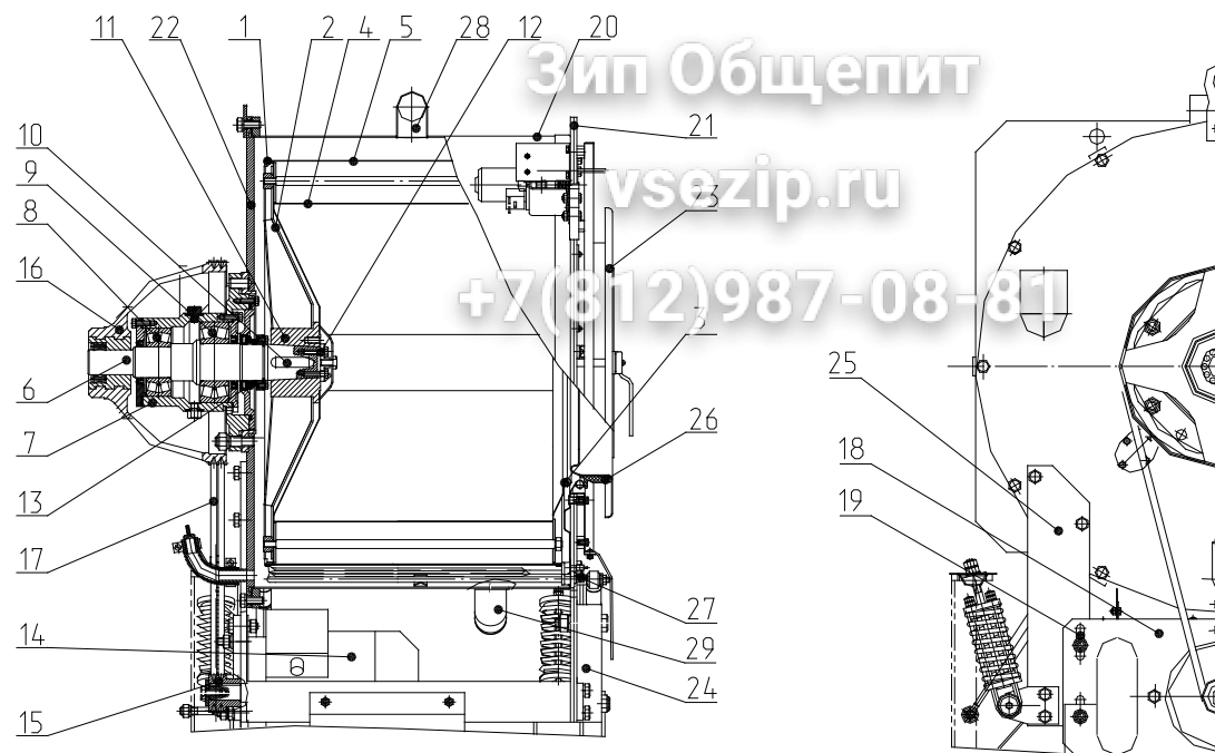
Рис.2 Блок барабанов
