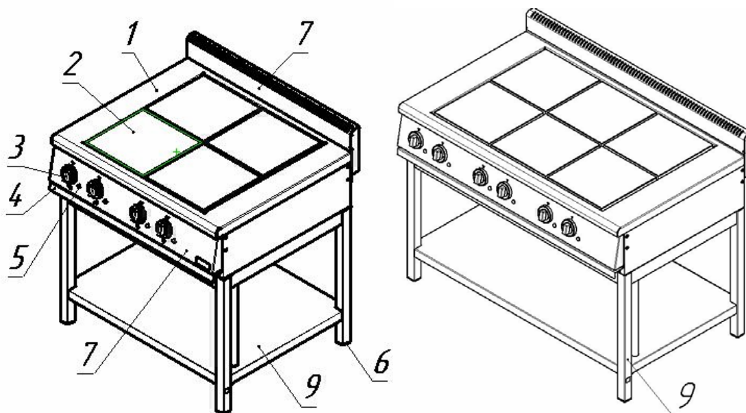
Рисунок 1- Составные части плит
