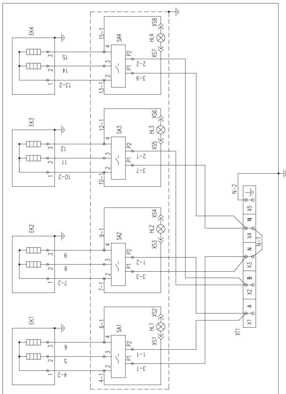
Рисунок 5-Схема электрическая принципиальная плиты ПЭ-724 О
