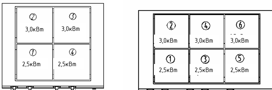
Рисунок 2 –Схема расположения конфорок
