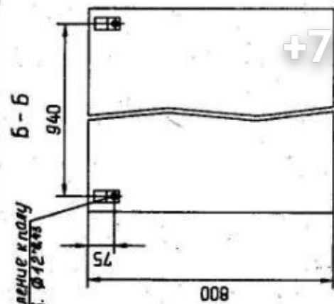
Схема крепления плиты к полу
