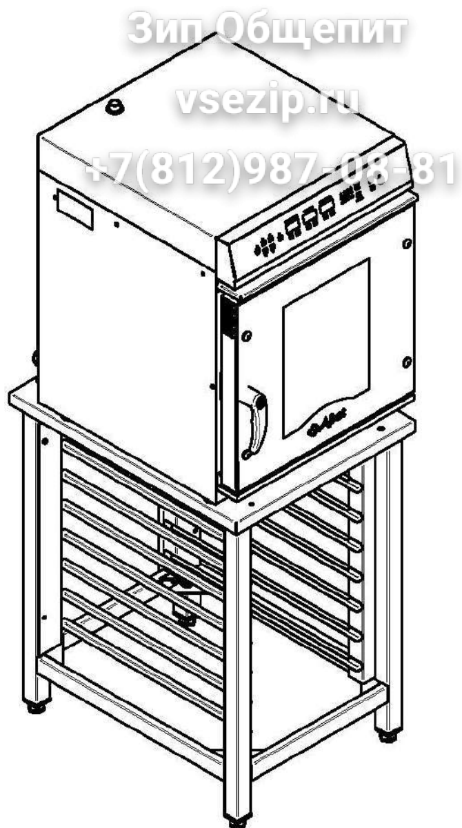
Рис.5. Пароконвектомат установленный на подставку ПК-8-02.
