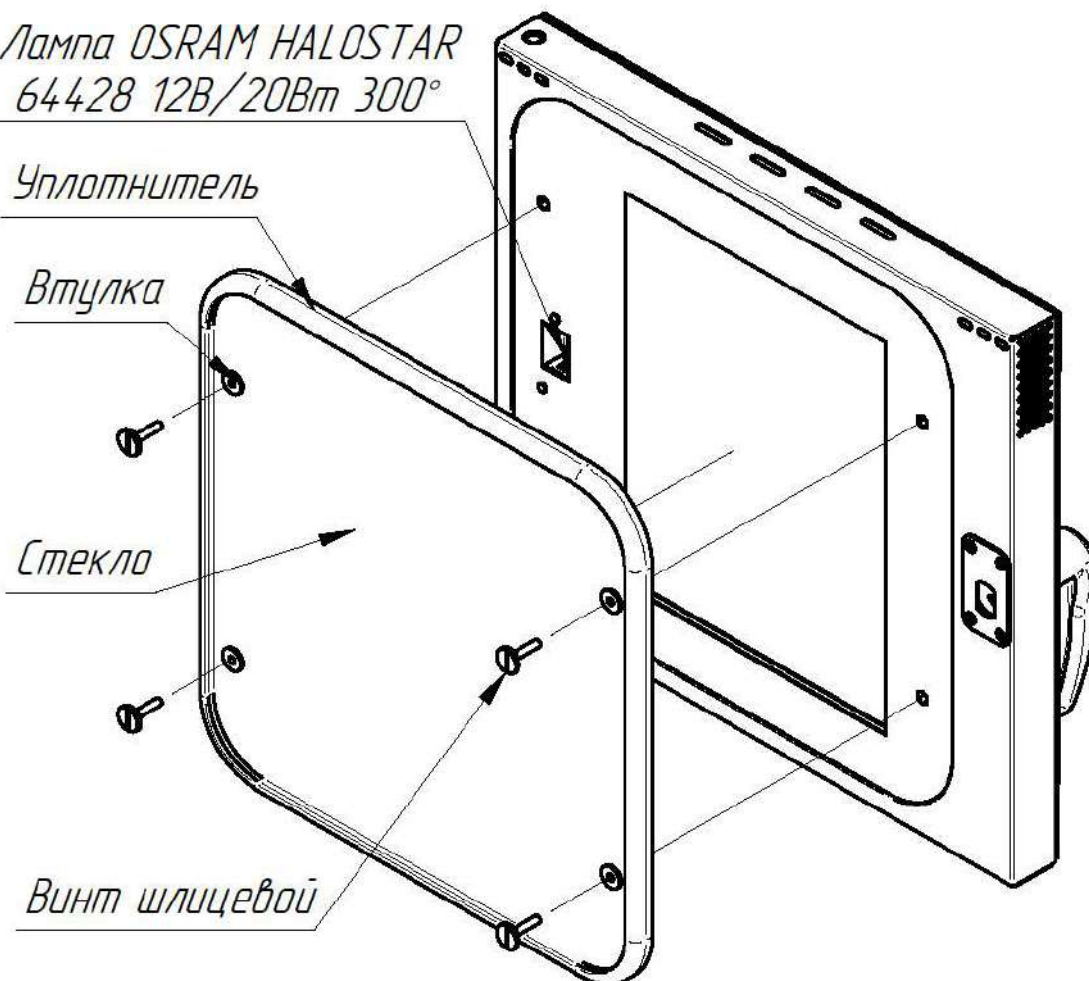
Рис.8. Замена лампы освещения и уплотнителя двери.
