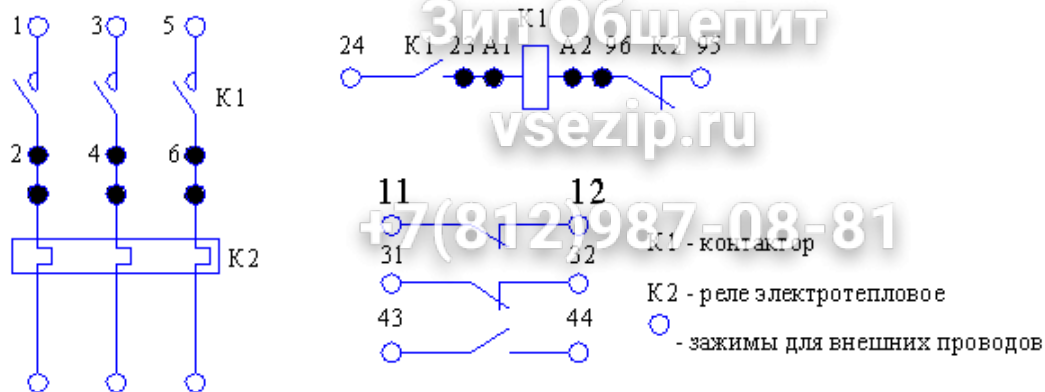
Рис. 2.73 - Пускатели неререверсивные с реле типа ПМЕ-212, ПМЕ-222, ПМА-3200, ПМА-3210
