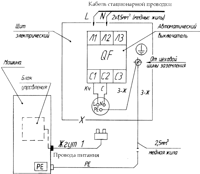
Рисунок 10 - Схема электрическая подключения мясорубки МИМ-80
