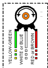
POTENTIOMETER 5÷10 kOhm
