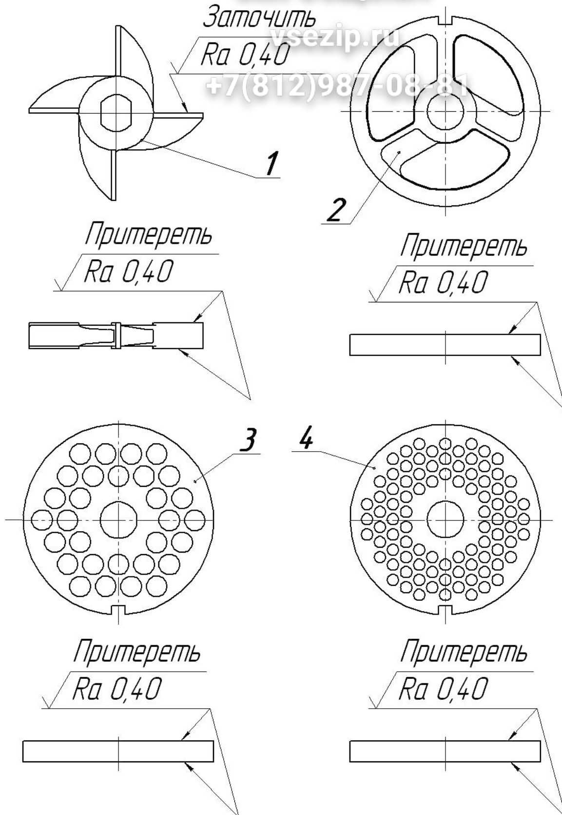
Рисунок 8 – Нож и решетки мясорубки ММП-ИИ-1
