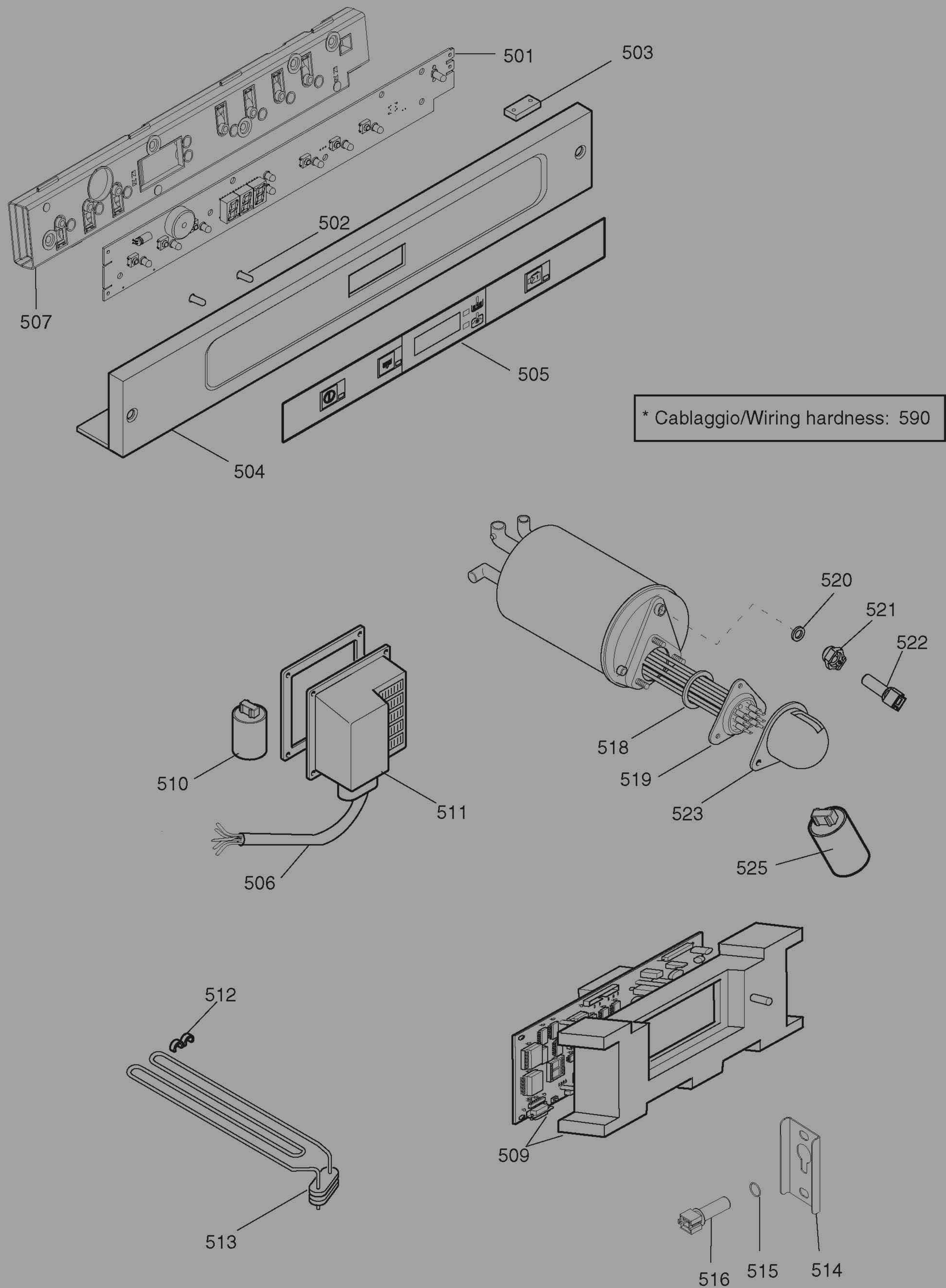
ill. 611002p5 Componenti elettrici / Electrical components
