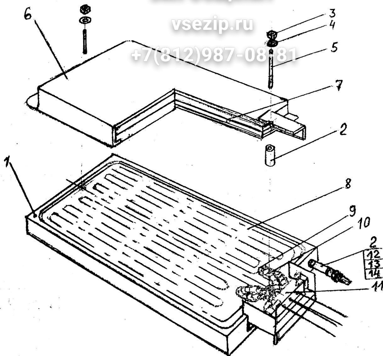
Рис. 16 ПЭ-0,48Ш.00.670
