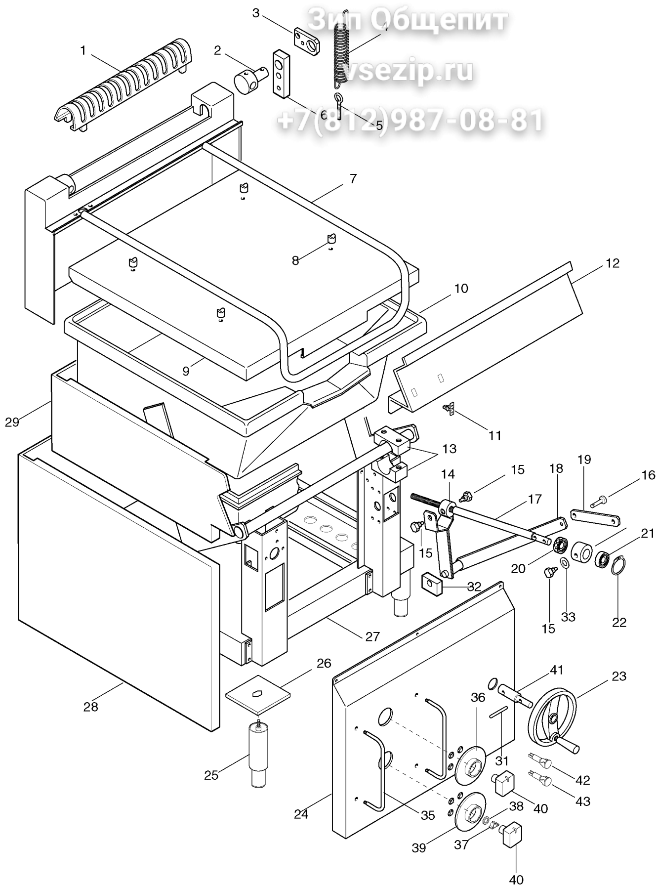
Brasiera Elettrica N700 Electric Bratt-Pan N700
