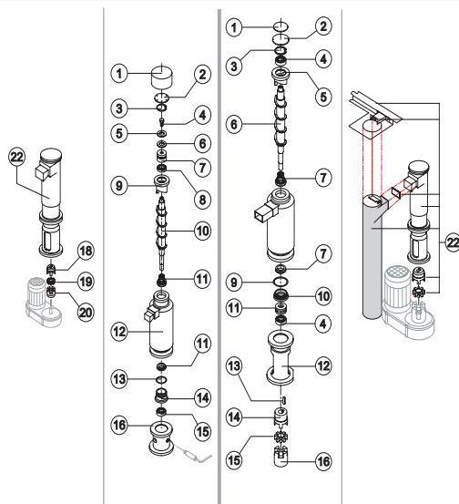
EVAPORATOR
