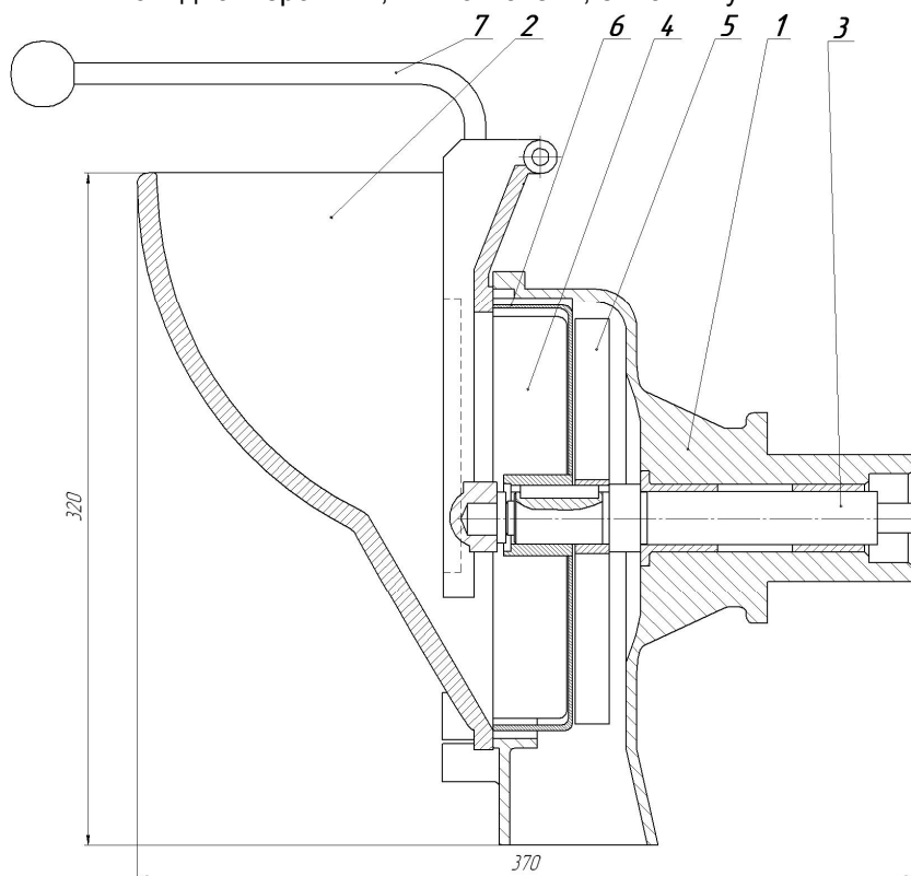
Рисунок 32 – Протирачный механизм, механизма МО –1
