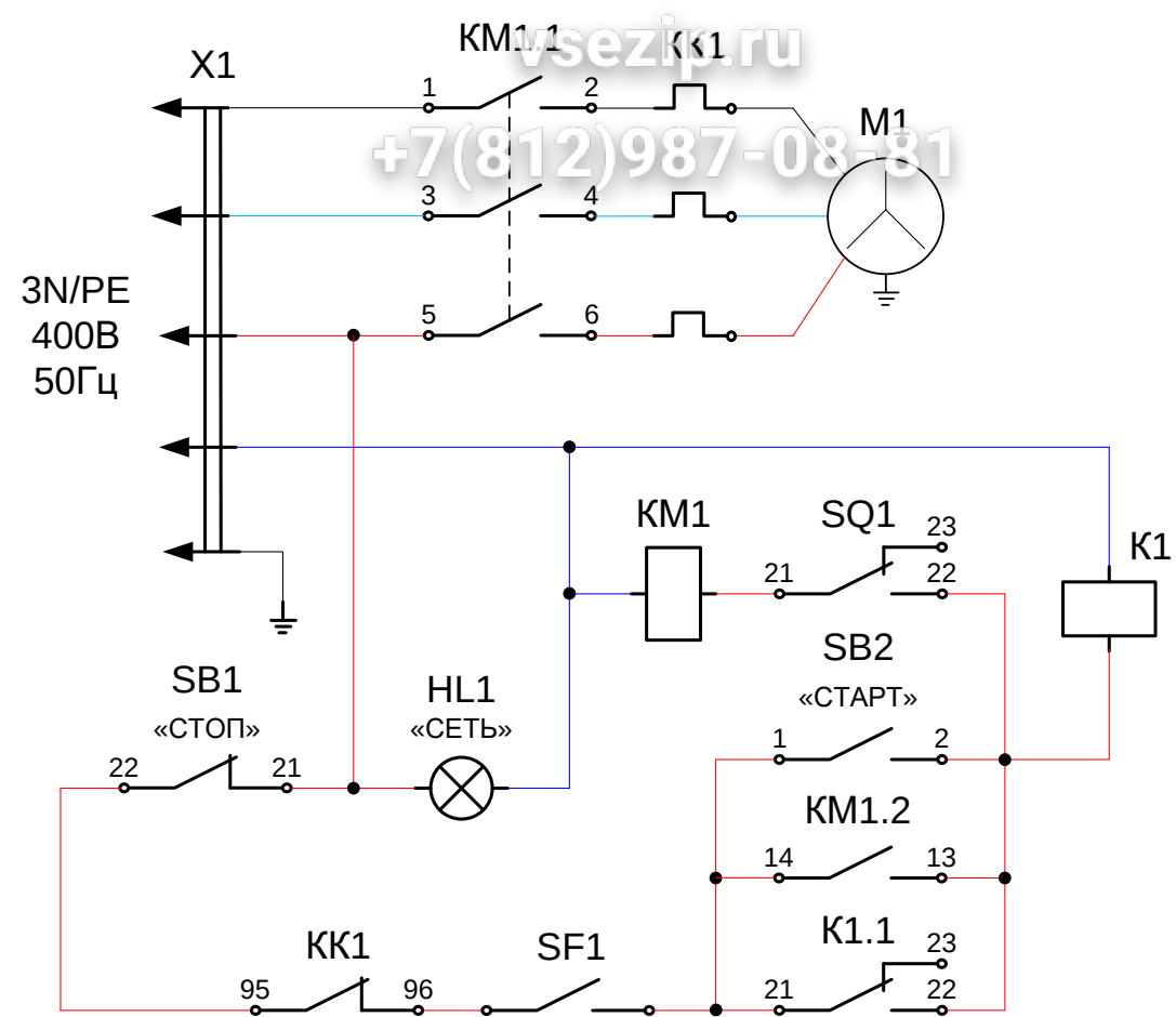
Схема электрическая принципиальная МКО-50
