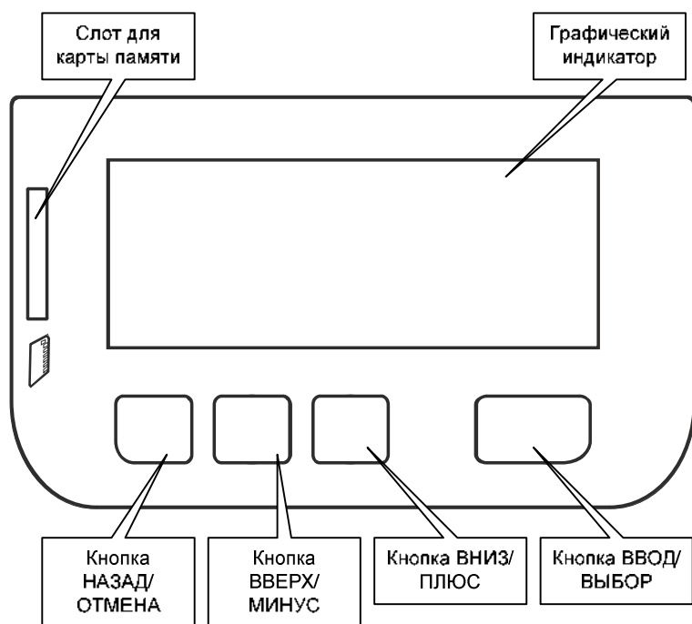
Лицевая панель контроллера, назначение кнопок
