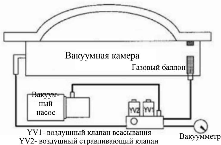
Схема вакуумного упаковщика с производительностью вакуумного насоса 10 мз
