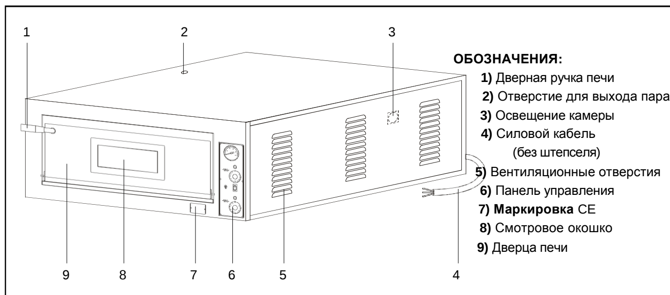
РИС.2 (Обозначение компонентов)
