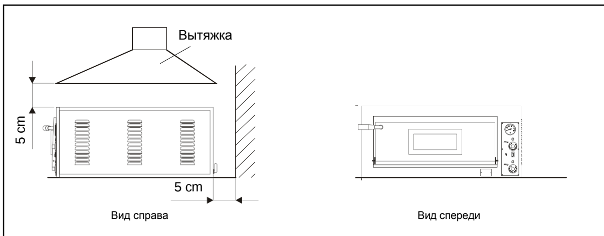
РИС.5 (Размещение)
