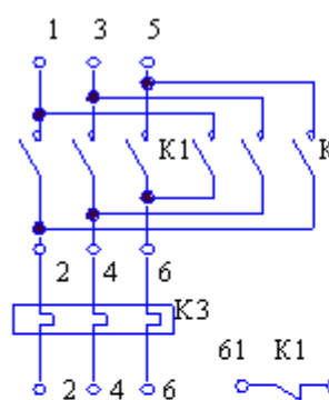
д) Пускатели типа ПМ12-025631, ПМ12-025671
