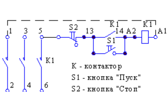
Рис. 2.3 - Пускатели нереверсивные без реле со встроенными в оболочку кнопками управления типа ПМ12-010160, ПМ12-010120 (1"з")
