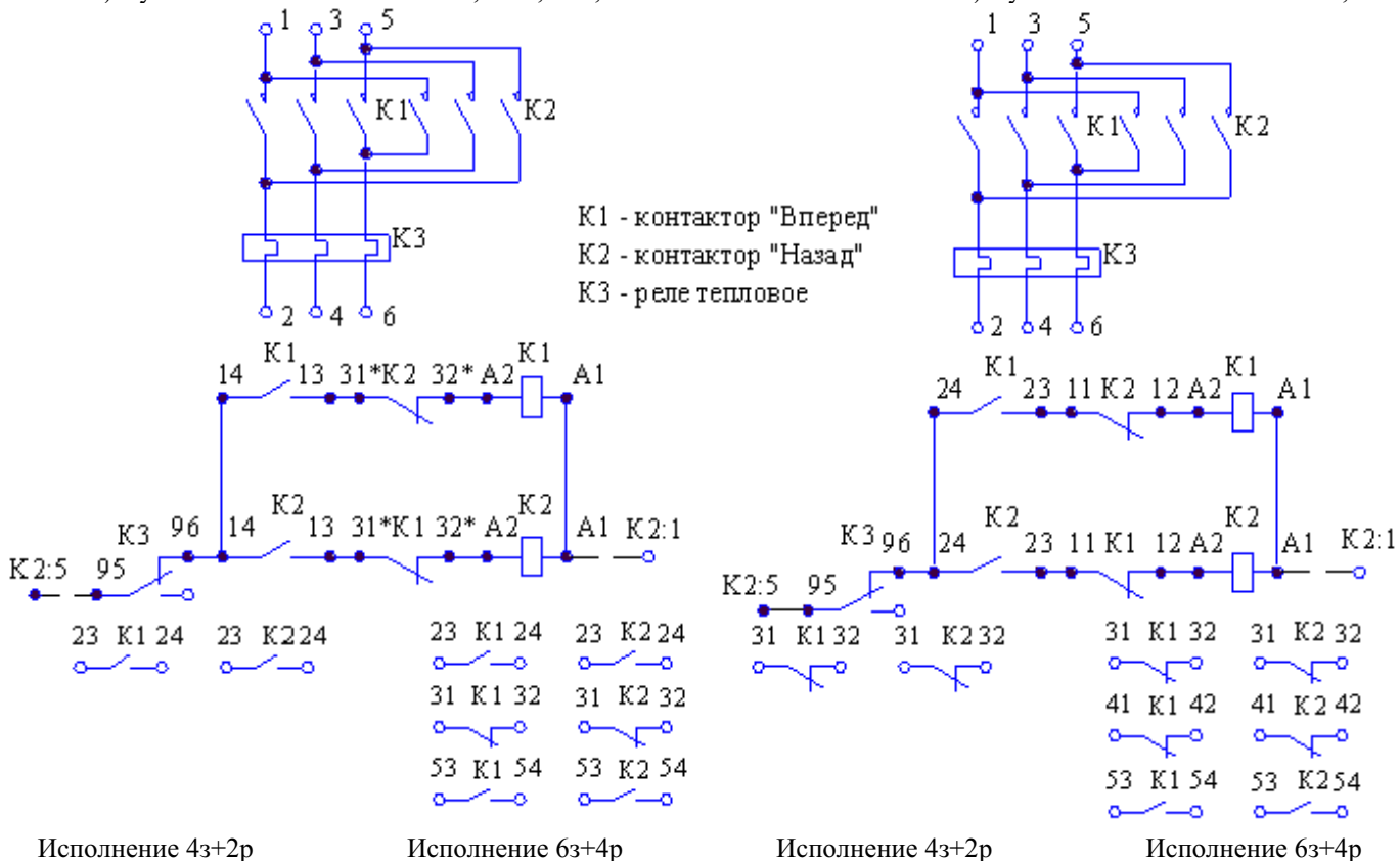
Рис. 2.7 - Пускатели реверсивные без реле, без кнопок управления типа ПМ12-010500, ПМ12-010550, ПМ12-010540, ПМ12-010510
