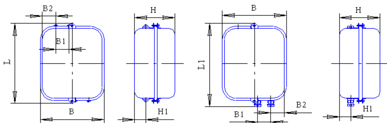
Рис. 2.36 – Пускатели реверсивные типа ПМ12-010600, ПМ12-010601, ПМ12-010650, ПМ12-010651
