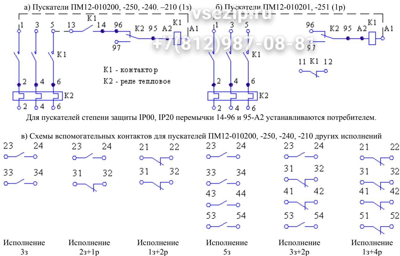
Рис. 2.2 - Пускатели нереверсивные с реле, без кнопок управления типа ПМ12-010 степени защиты IP00, IP20, IP40, IP54
