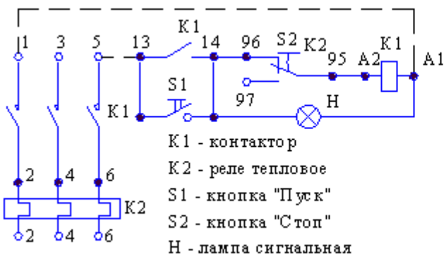
Рис. 2.5 - Пускатели нереверсивные со встроенными в оболочку кнопками управления и сигнальной лампой типа ПМ12-010270, ПМ12-010230 («1з»)
