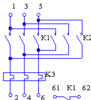
в) Пускатели типа ПМ12-025611, ПМ12-025641
