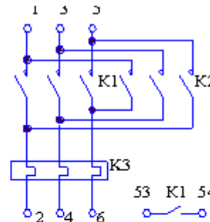
г) Пускатели типа ПМ12-040610, ПМ12-040640
