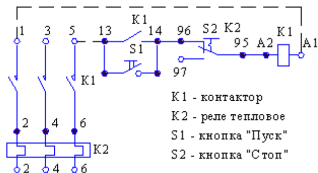
Рис. 2.4 - Пускатели нереверсивные с реле со встроенными в оболочку кнопками управления типа ПМ12-010260, ПМ12-010220 (1"з")
