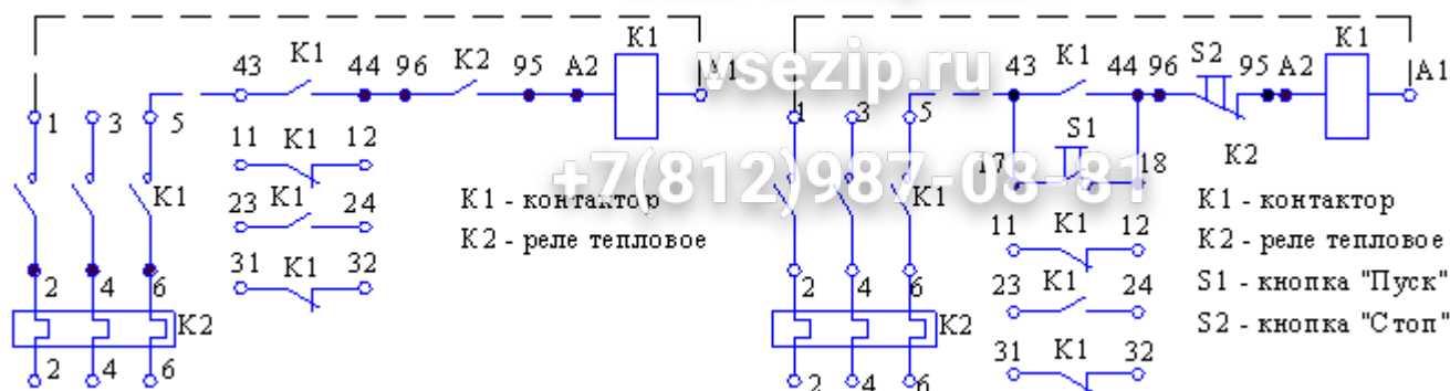
Рис. 2.27 – Пускатели неперевсивные с реле типа ПМ12-063 в оболочках степени защиты IP40, IP54
