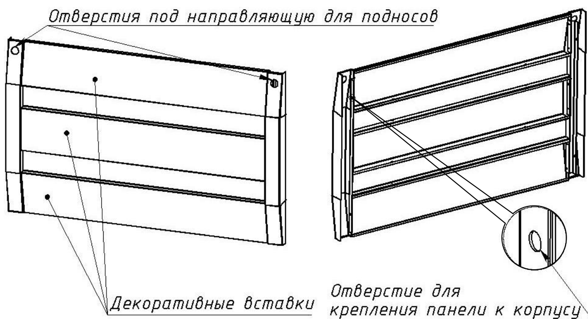
Рис.5 Панель декоративная.
