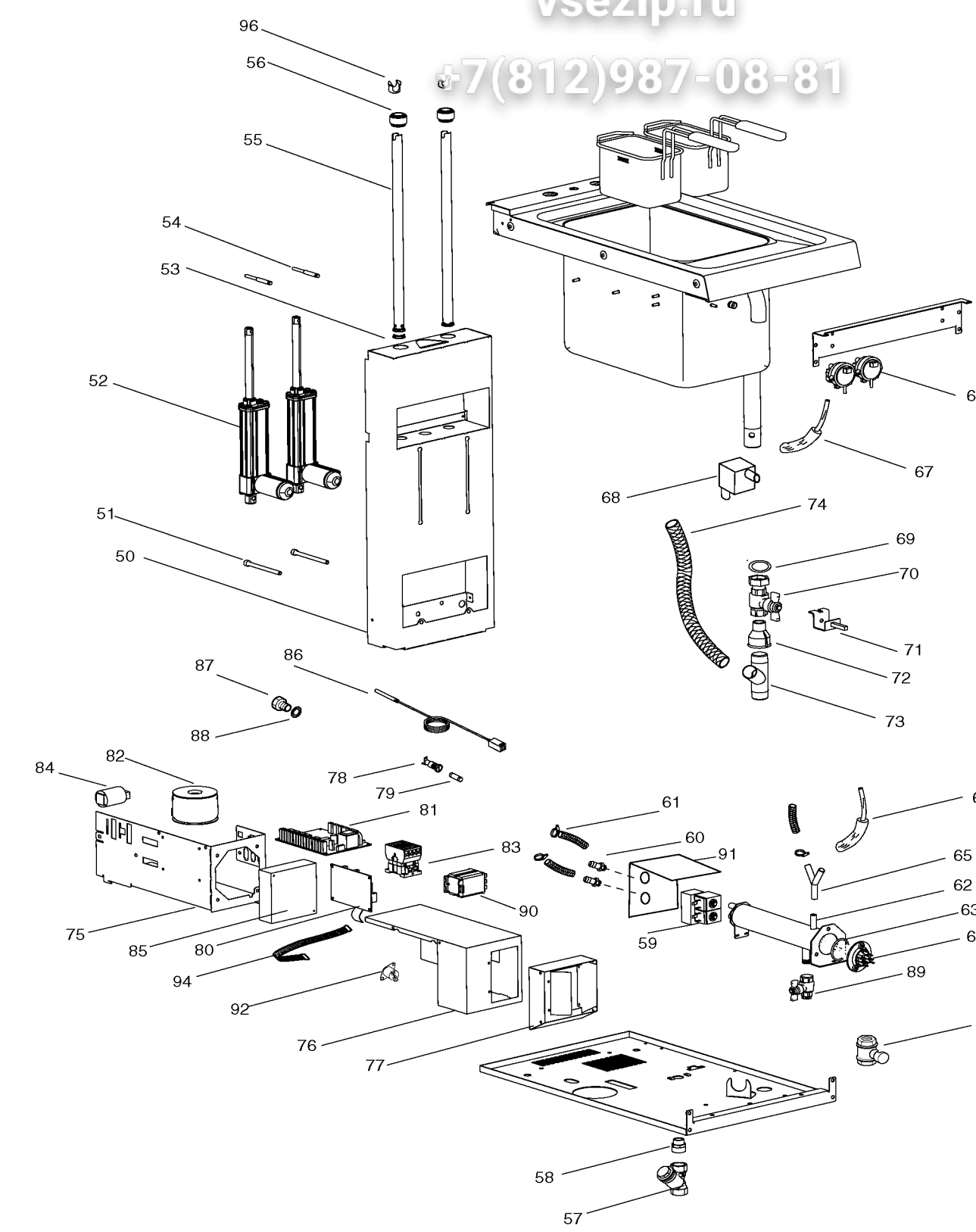
Cuocipasta elettrico automatico elettronico N700 Electric automatic electronic Pasta cooker N700
