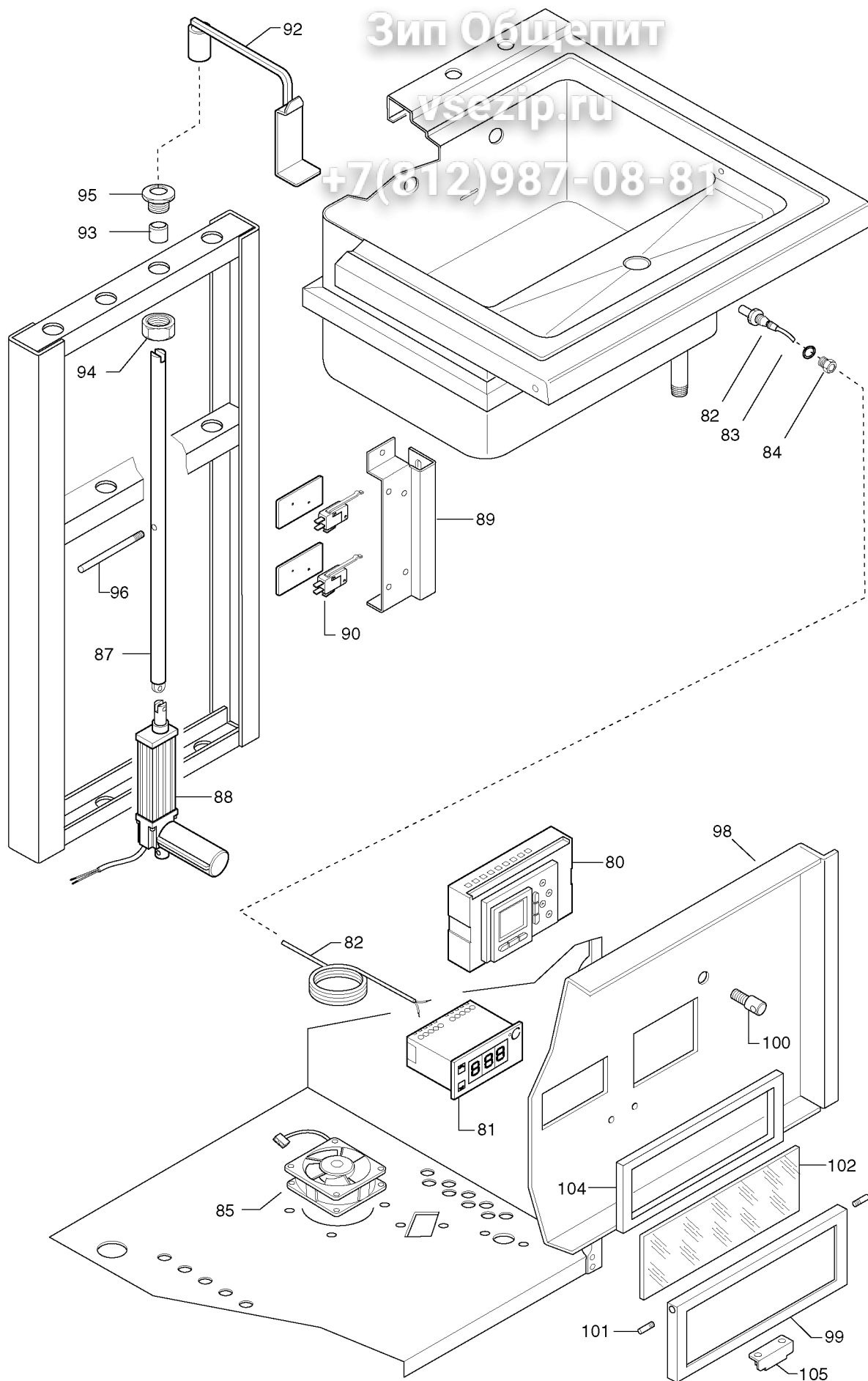
AUTOMATIC ELECTRIC PASTA COOKER PR700 CUOCIPASTA ELETTRICO AUTOMATICO PR700
