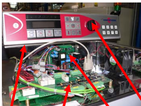
Стандартная панель управления ST5020 с кнопками и поворотным регулятором
