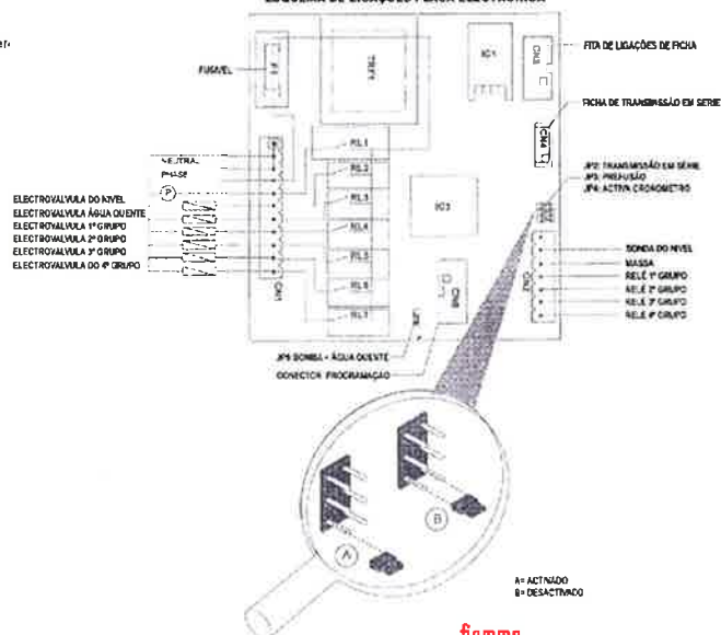
ESQUEMA DE LIGAÇÕES PLACA ELECTRÓNICA
