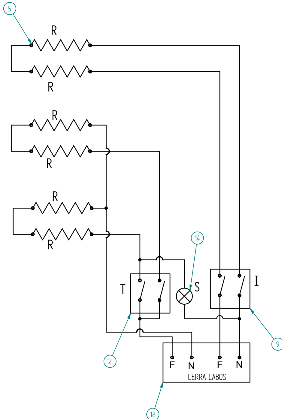
ESQUEMA ELECTRICO
