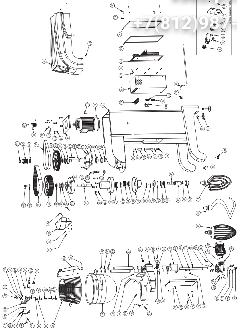
FIG. / РИС. 32 - MX40/60/80 TV Parti di ricambio / Replacement parts / Pieces de rechange / Repuestos / Запасные части
