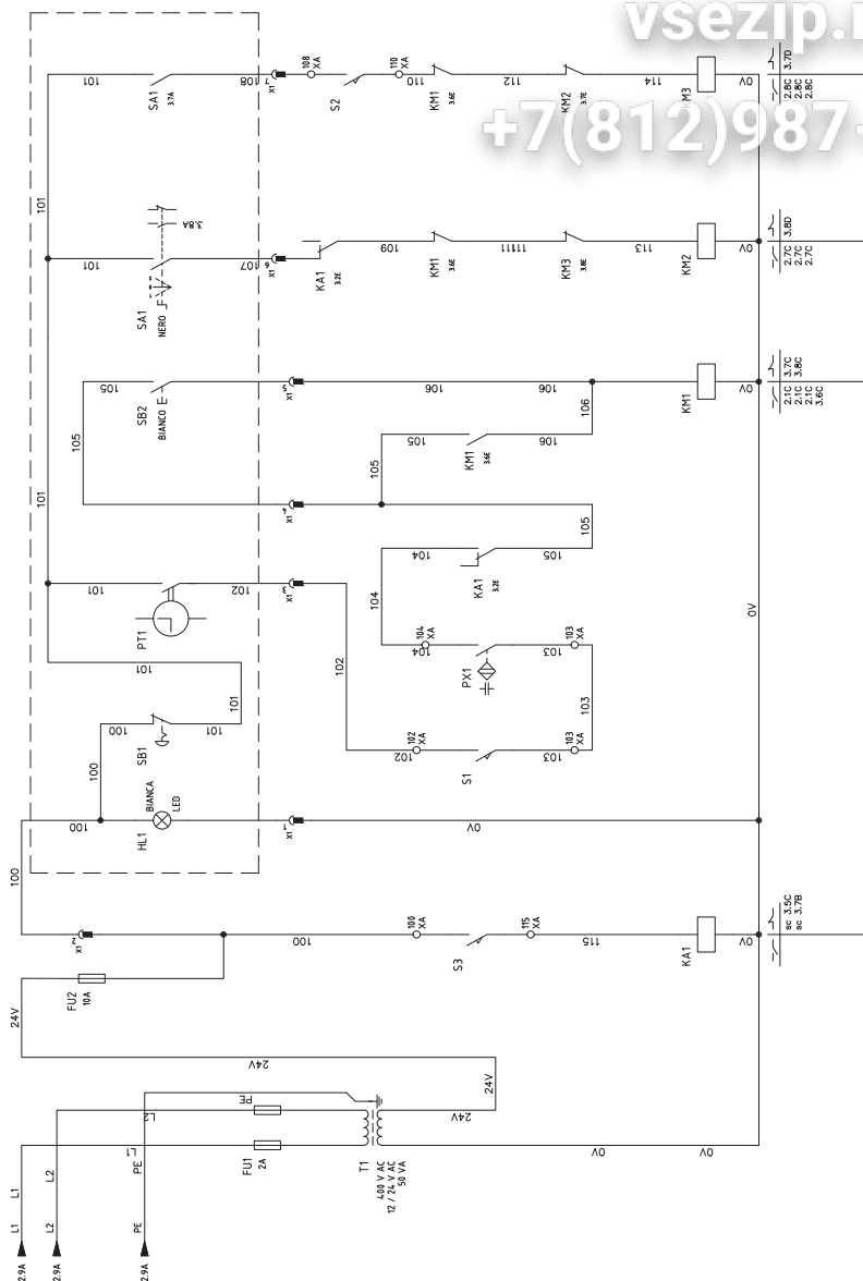
FIG. / PИC. 17 - MX40/60/80 TV Schema elettrico / Electrical diagram / Schémas électriques / Diagrama eléctricos / Монтажная схема
