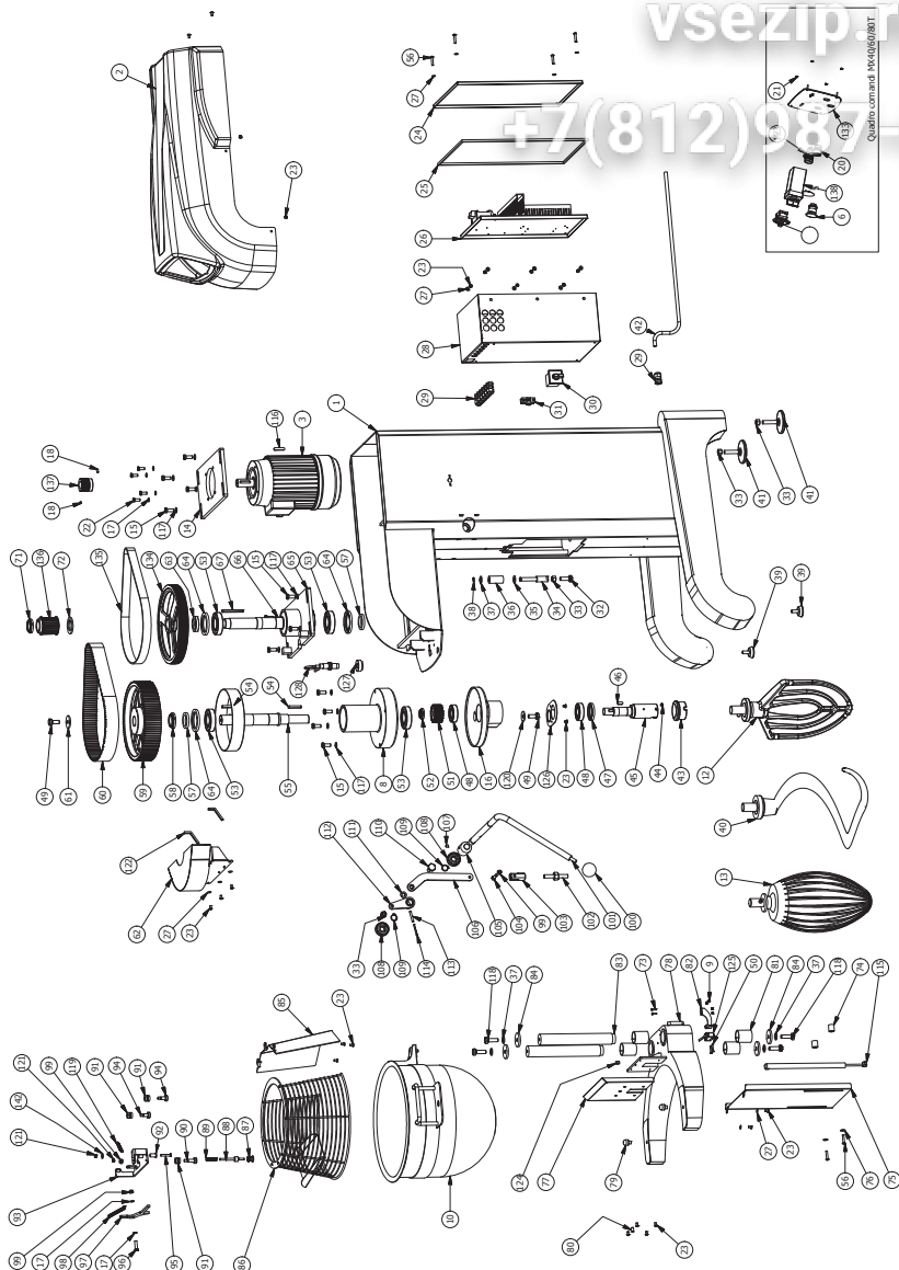
FIG. / РИС. 31 - MX40/60/80 T Parti di ricambio / Replacement parts / Pieces de rechange / Repuestos / Запасные части
