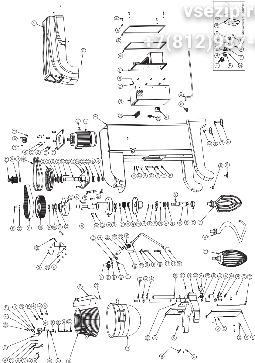
FIG. / РИС. 34 - MX40/60/80 P Parti di ricambio / Pieces de rechange / Repuestos / Запасные части
