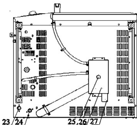
Рис.1. Пароконвектомы «Рубикон» АПК6-1/1 и АПК10-1/1.
