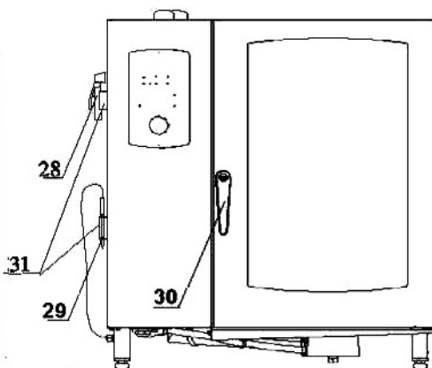
Рис.1. Пароконвектомы «Рубикон» АПК6-1/1 и АПК10-1/1.
