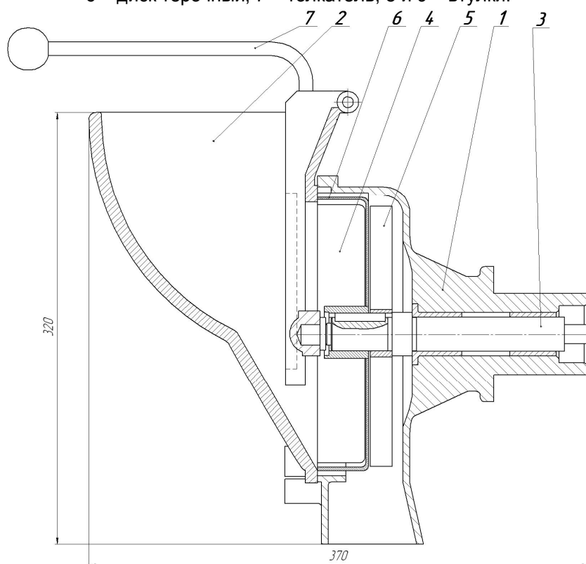
Рисунок 32 – Протирающий механизм, механизма МО –1
