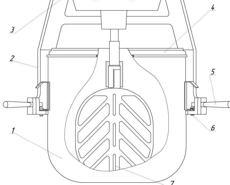
Рисунок 6 – Механизм для взбивания и перемешивания ВМ
