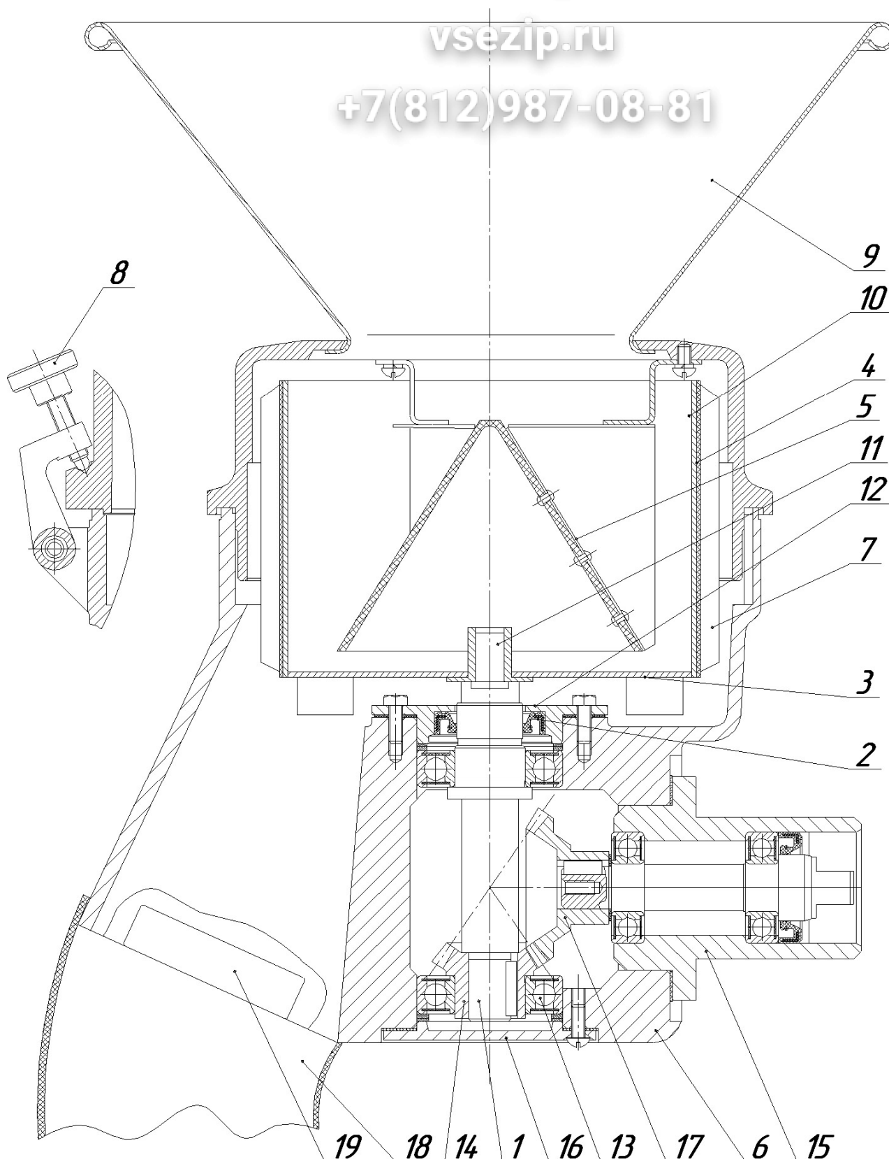
Рисунок 19 – Росеиватель МП – 01
