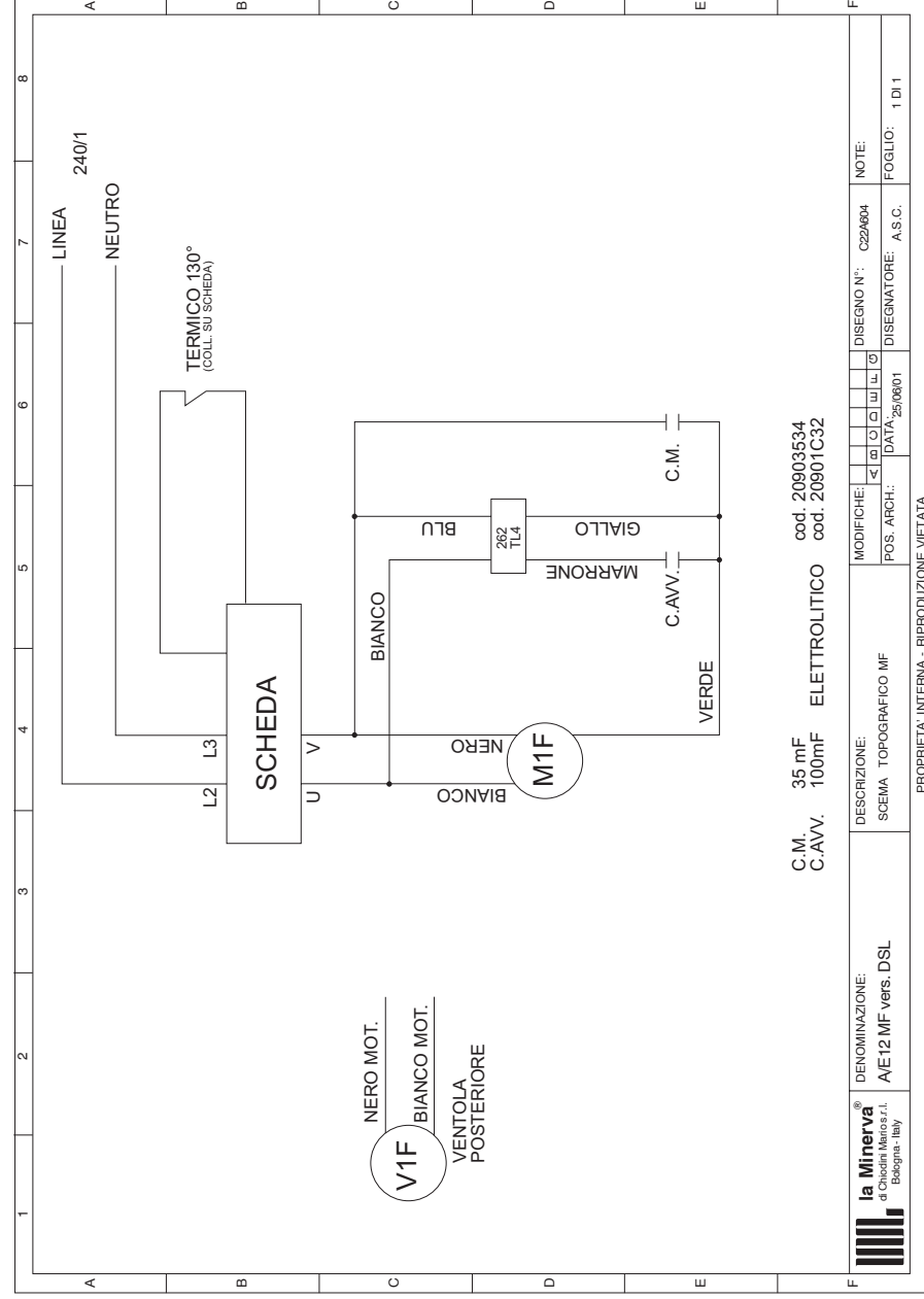
Schema Topografico MF / Layout MF / Schéma Topographique MF / Anschlussplan MF / Esquema Topográfico MF
