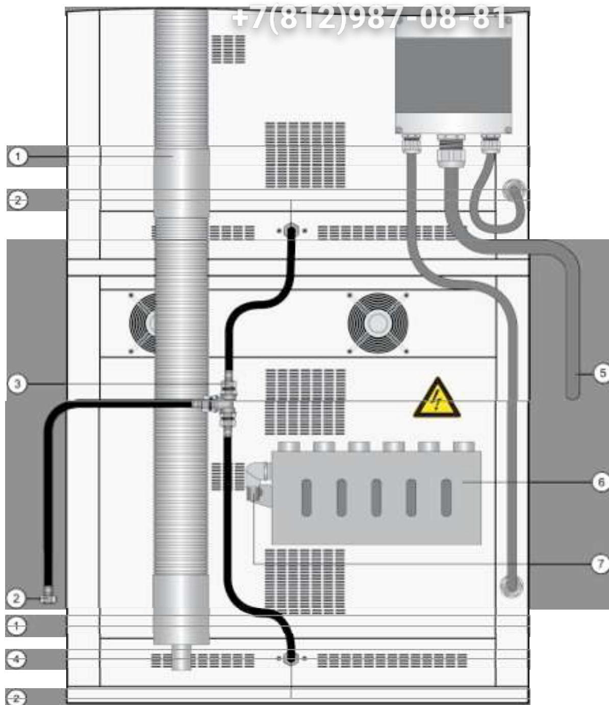
Рис. 1 Подключения с задней стороны установки MIWE econo 8.0604
