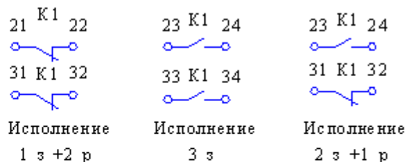
Рис. 2.4 - Пускатели нереверсивные с реле со встроенными в оболочку кнопками управления типа ПМ12-010260, ПМ12-010220 (1"з")
